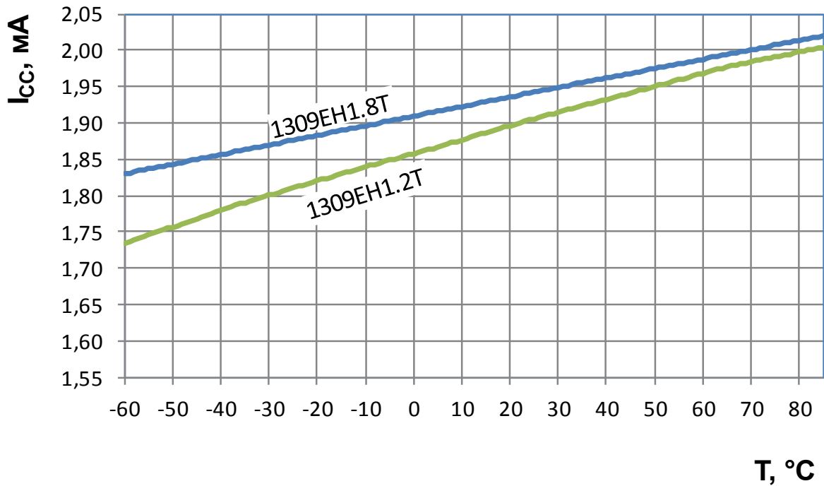
Рисунок 19 – Зависимость тока потребления I_{CC} от температуры при U_1 = 5,5 В, I_o = 10 мА
