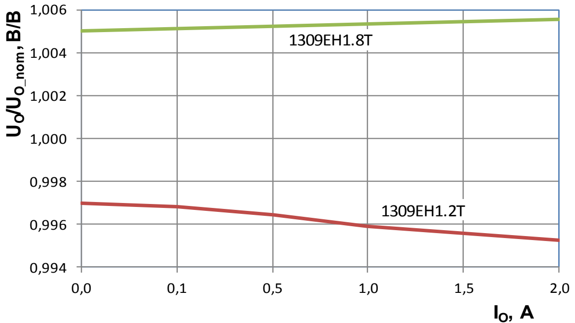
Рисунок 9 – Зависимость выходного напряжения U_o (приведенного к выходному напряжению номинальному U_{o\_nom} ) от тока нагрузки при U_i = 2,8 В для 1309ЕН1.2Т и U_i = 2,6 В для 1309ЕН1.8Т, T = 25 °С
